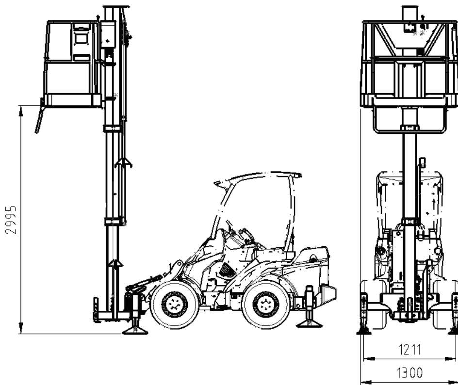
Obrázok 2 – Vysokozdvížná plošina Leguan 50 pripojená k nakladaču Avant
