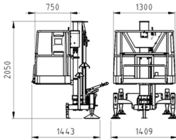
Obrázok 1 – Vysokozdvížná plošina Leguan 50 v prepravnej konfigurácii
